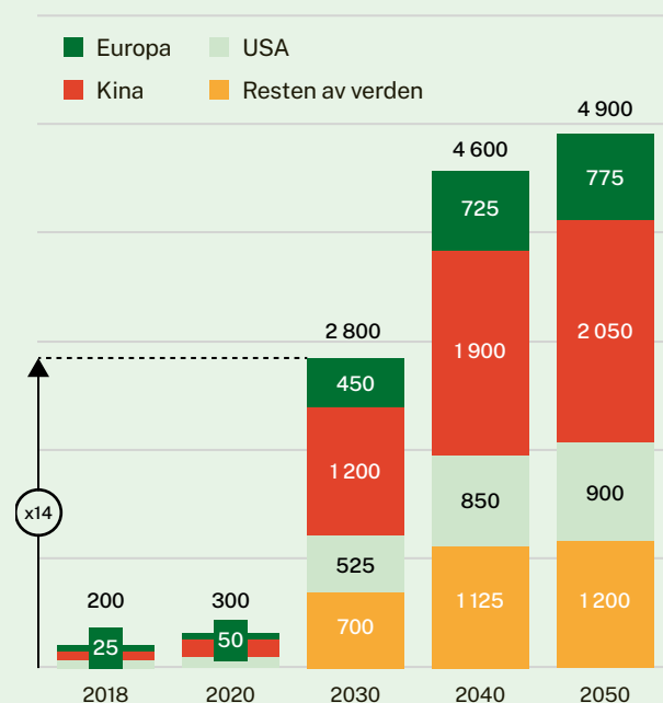
Global batterietterspørsel, GWh
