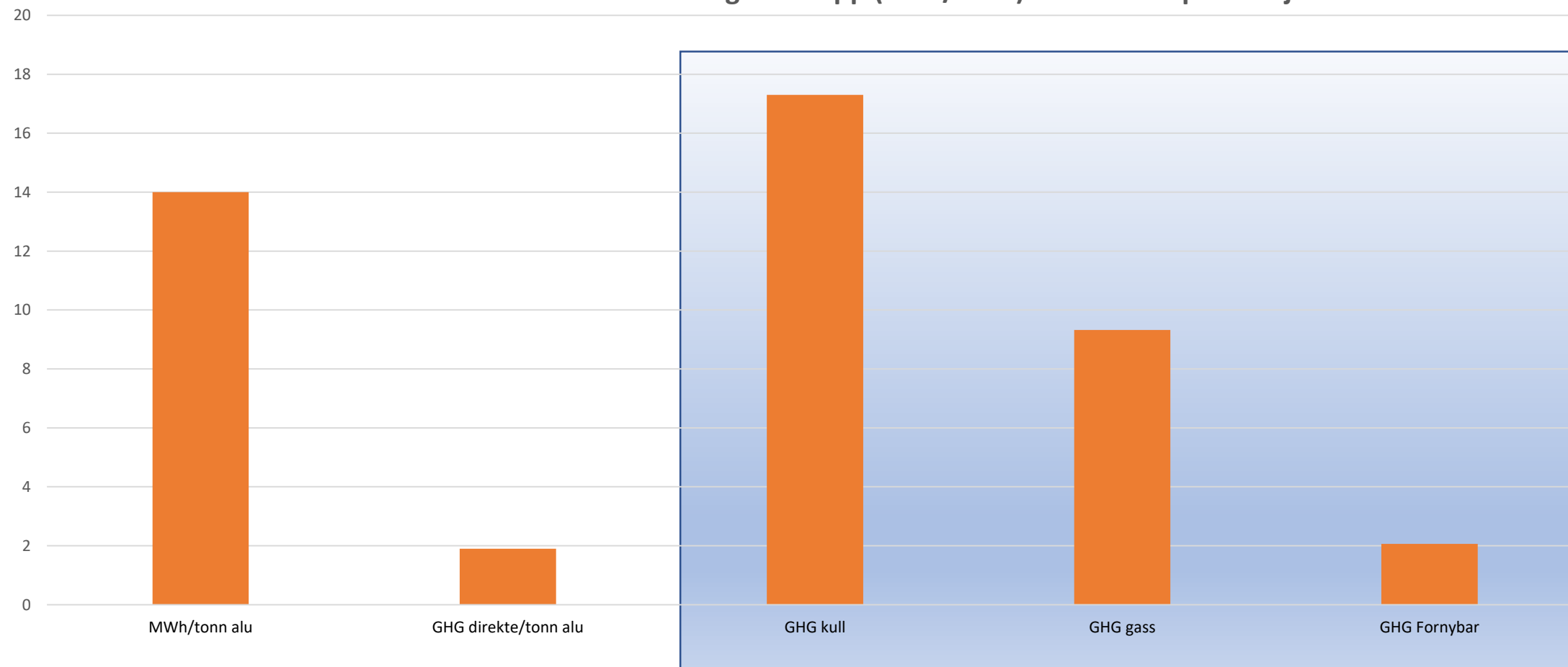
Klimagassutslipp (tonn/tonn) aluminiumsproduksjon med ulike kraftkilder
